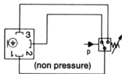
連接插頭接線圖 (ISO 4400) :
